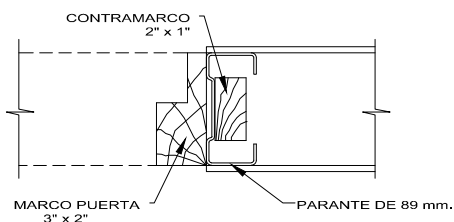
DETALLE
